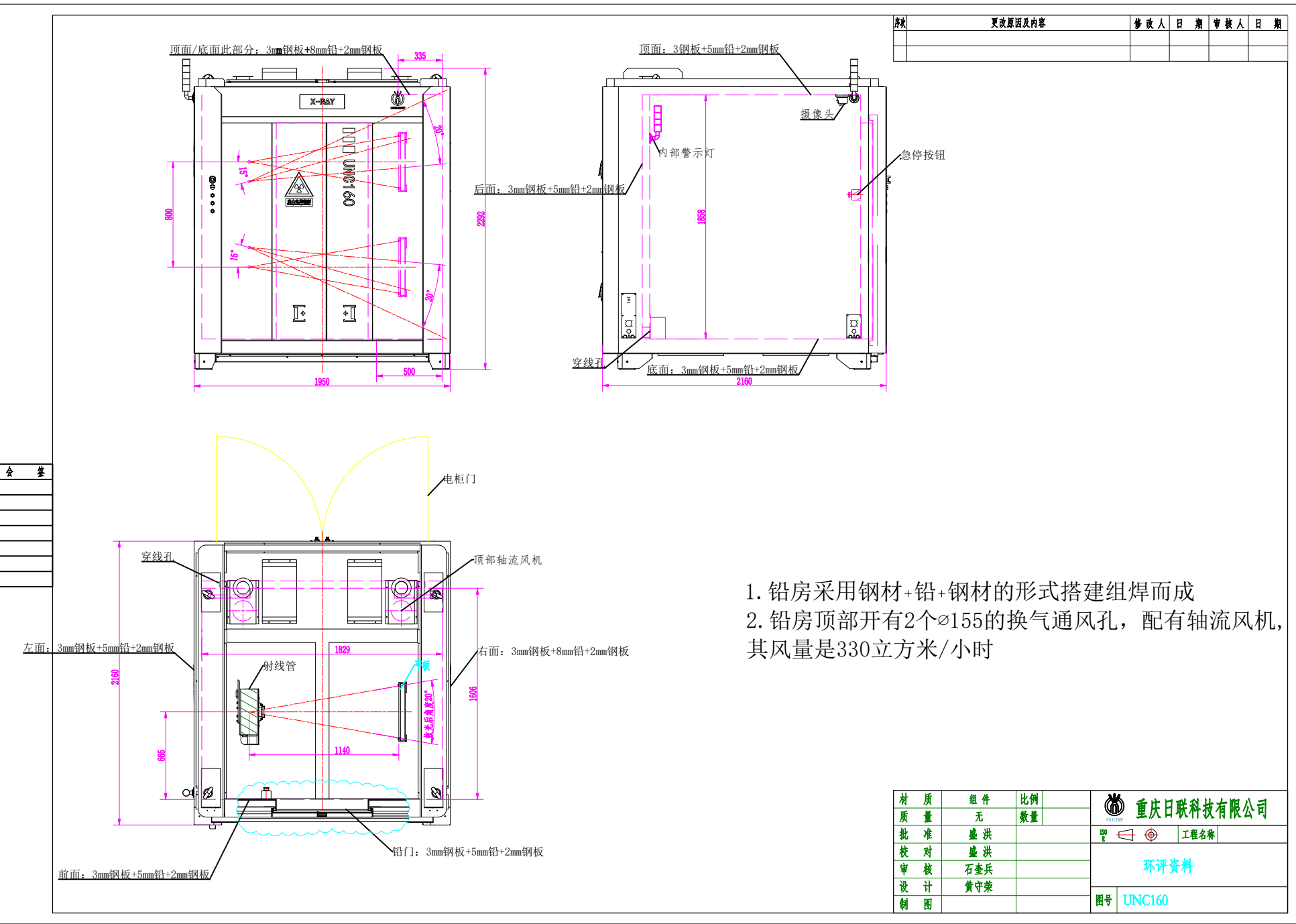
附图5 本项目X射线数字成像检测设备屏蔽设计图
