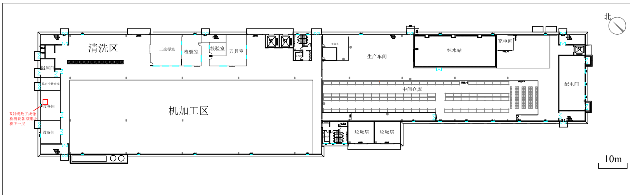
附图3-1 本项目装置所在厂房一层平面布置图
