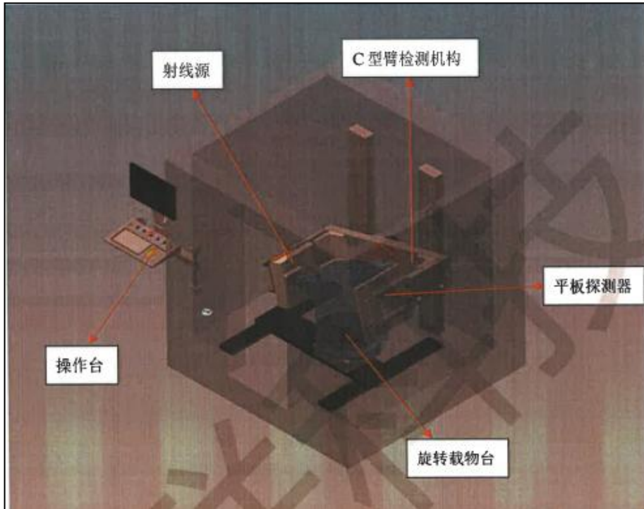
图 9-1 UNC160 型 X 射线数字成像检测设备示意图
