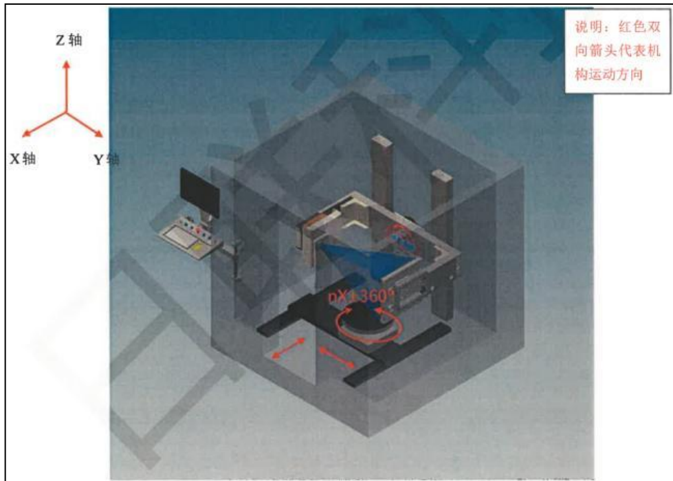
图 9-2 UNC160 型 X 射线数字成像检测设备内部载物台移动示意图
