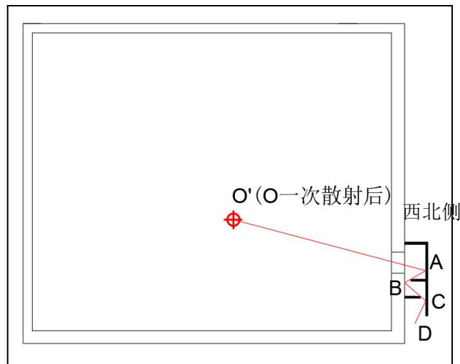
图 11-2 本项目电缆管道散射示意图
