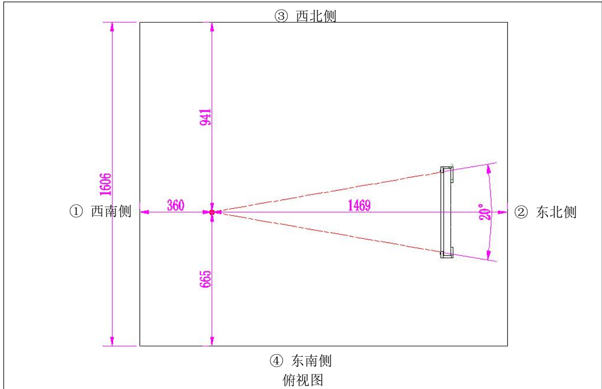
图 11-1 本项目 X 射线数字成像检测设备各关注点位示意图（单位：mm）
