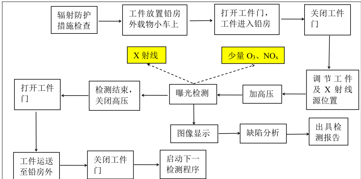
图 9-6 本项目 X 射线数字成像检测设备工作流程及产污环节
