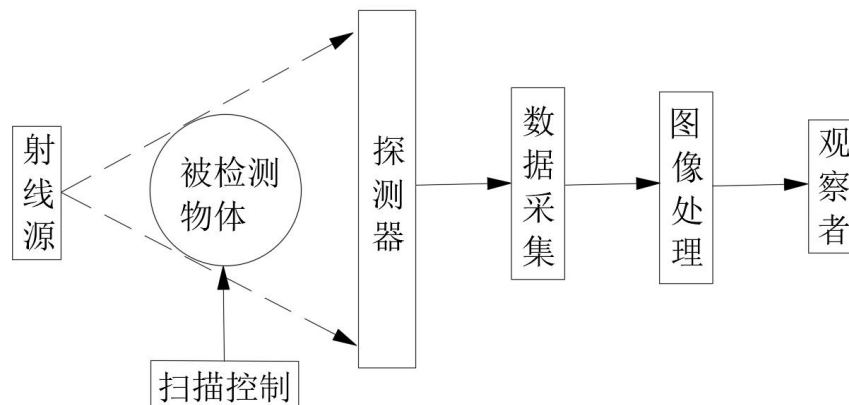
图 9-5 X 射线数字成像检测设备结构工作原理简图
