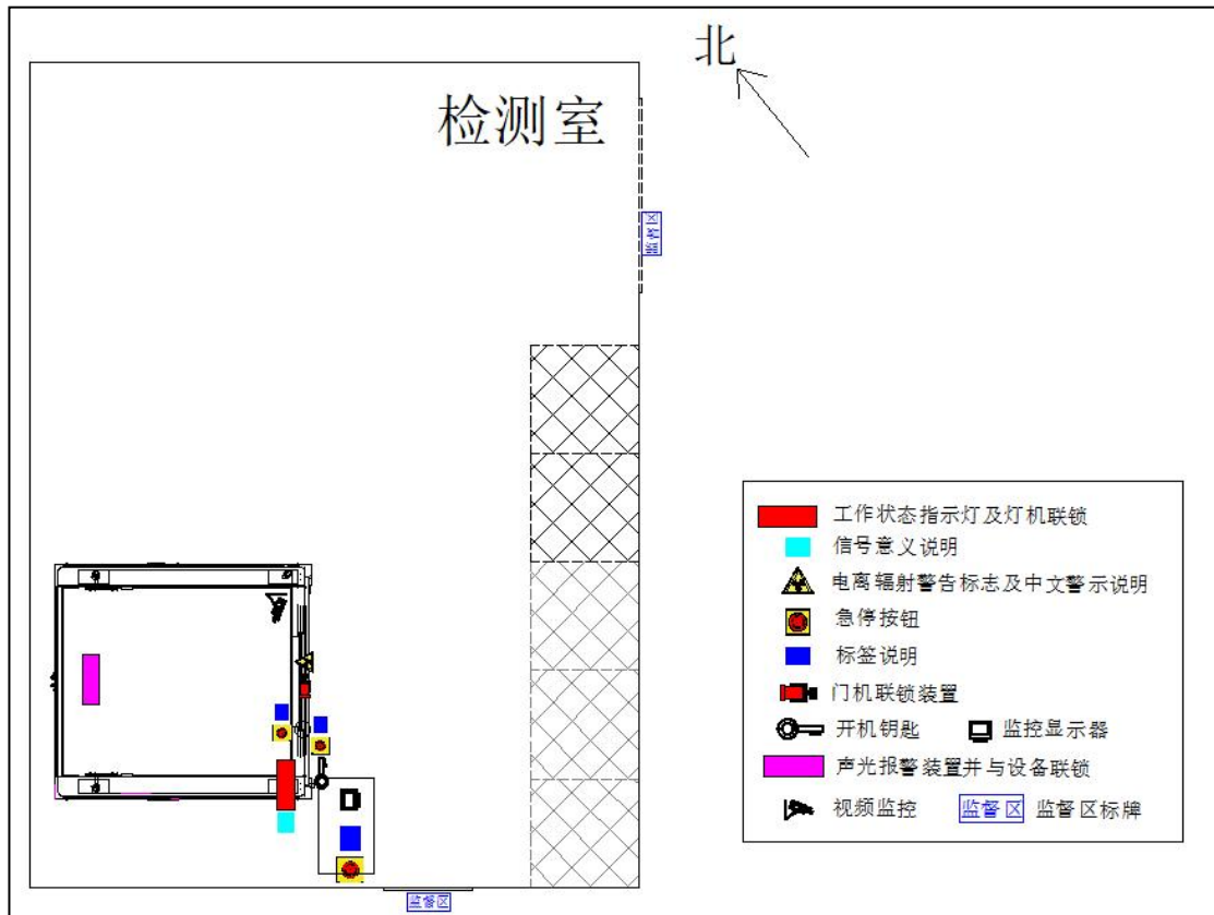
图 10-2 本项目辐射安全和防护措施示意图
