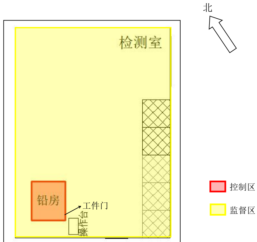
图 10-1 本项目 X 射线数字成像检测设备监督区及控制区示意图
